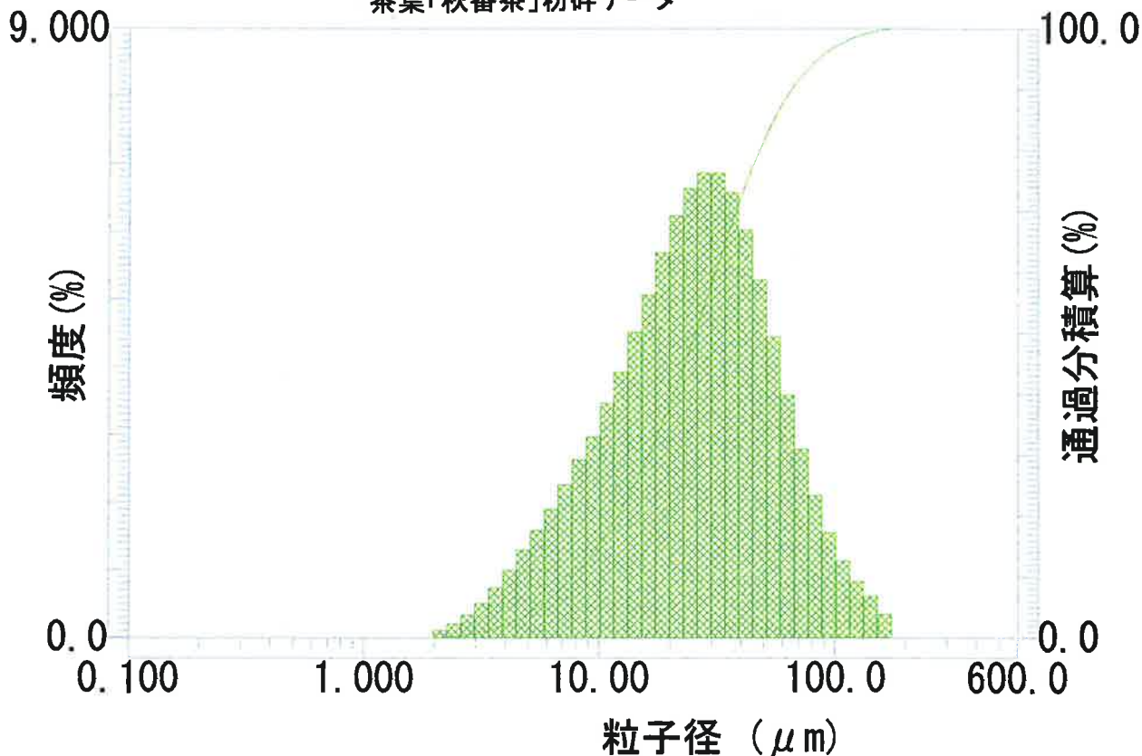
当社現行の低温微粉碎機にて加工 茶葉「秋番茶」粉碎データ
