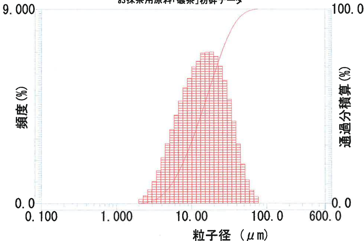
当社現行の低温微粉碎機にて加工 お抹茶用原料「碾茶」粉碎データ
